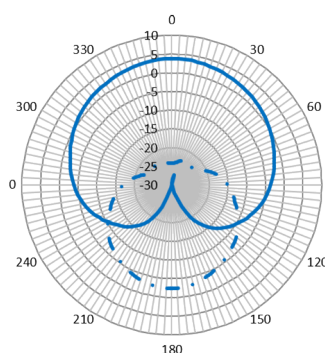
Vertical (ETSI)
