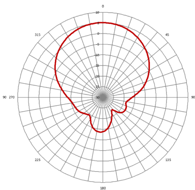
Vertical (ETSI)
