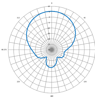
Horizontal (ETSI)
