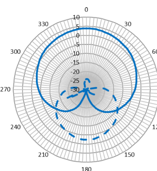
Horizontal (ETSI)
